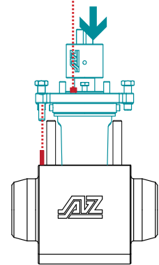
Montage der neuen Kartusche (codierte Einbaulage)
