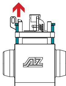
Anheben der Kartusche mit zwei Abziehschrauben
