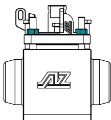
Lösen der Deckelschrauben
