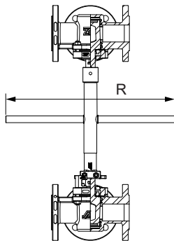
Typ UK mit T-Hebel
