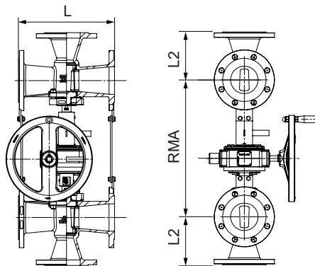
Typ UK mit Handgetriebe
