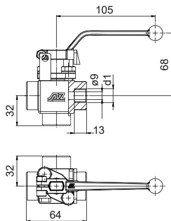
Typ MGZ-24 mit Innengewinde
