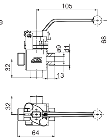
Typ MGZ-24 mit Außengewinde
